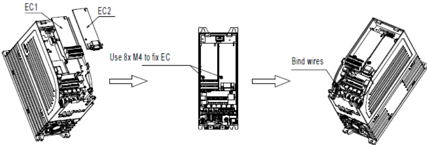
Рис А-1 ПЧ 1,5 – 7,5 кВт с установленными платами расширения
