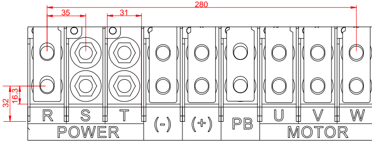
Рис. 4-26 Клеммы силовых цепей 110–132 кВт (единица измерения: мм)
