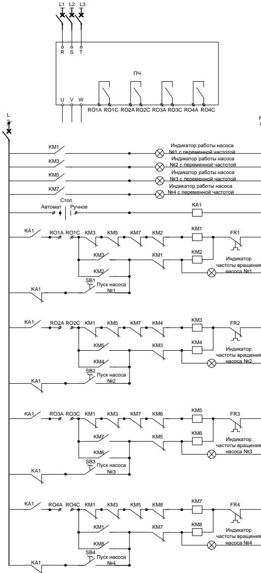
Рис. 5–3 Схема подключения цепей управления
